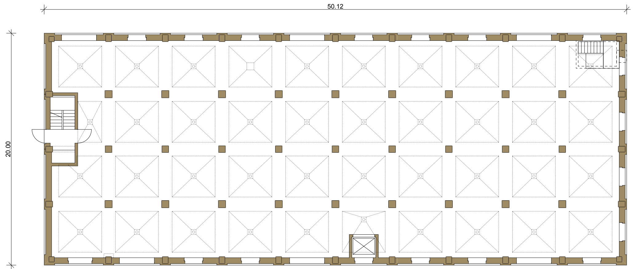
Erdgeschoss Silohalle (Hochparterre) (±0.00)
