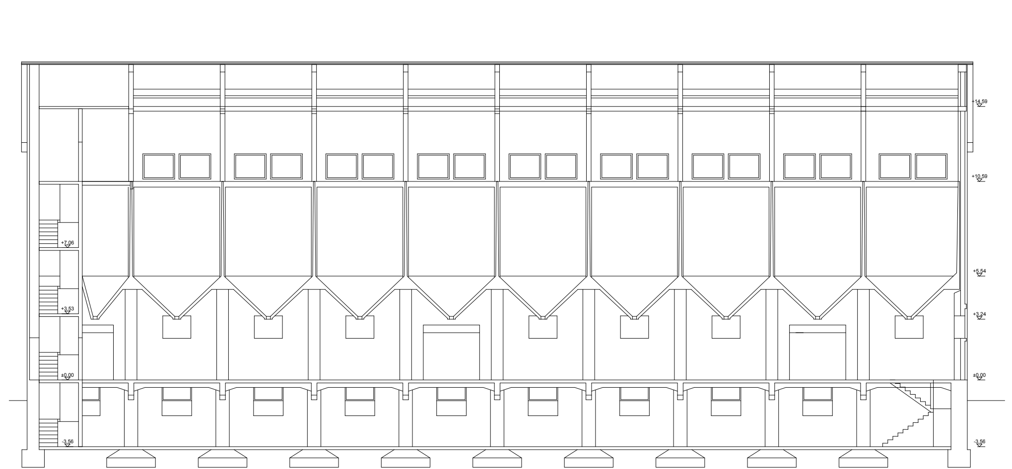
Längsschnitt Silogebäude
