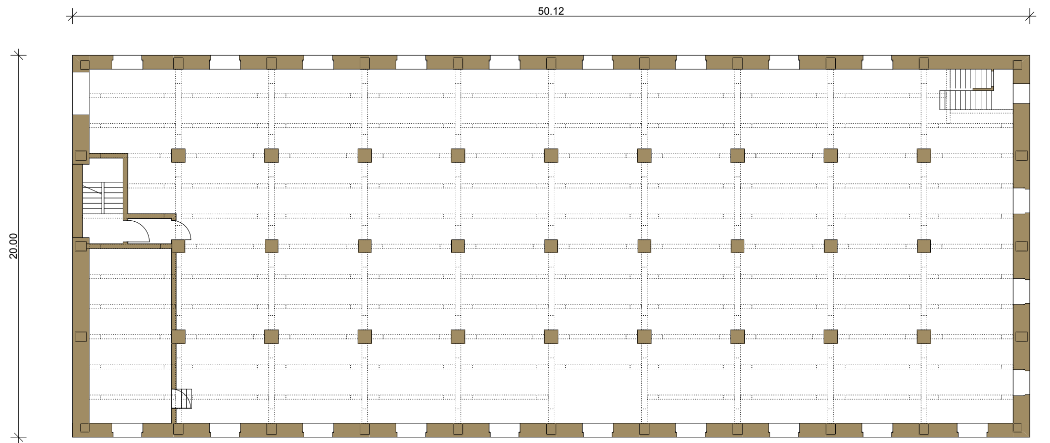
Untergeschoss Silogebäude (-3.56)
