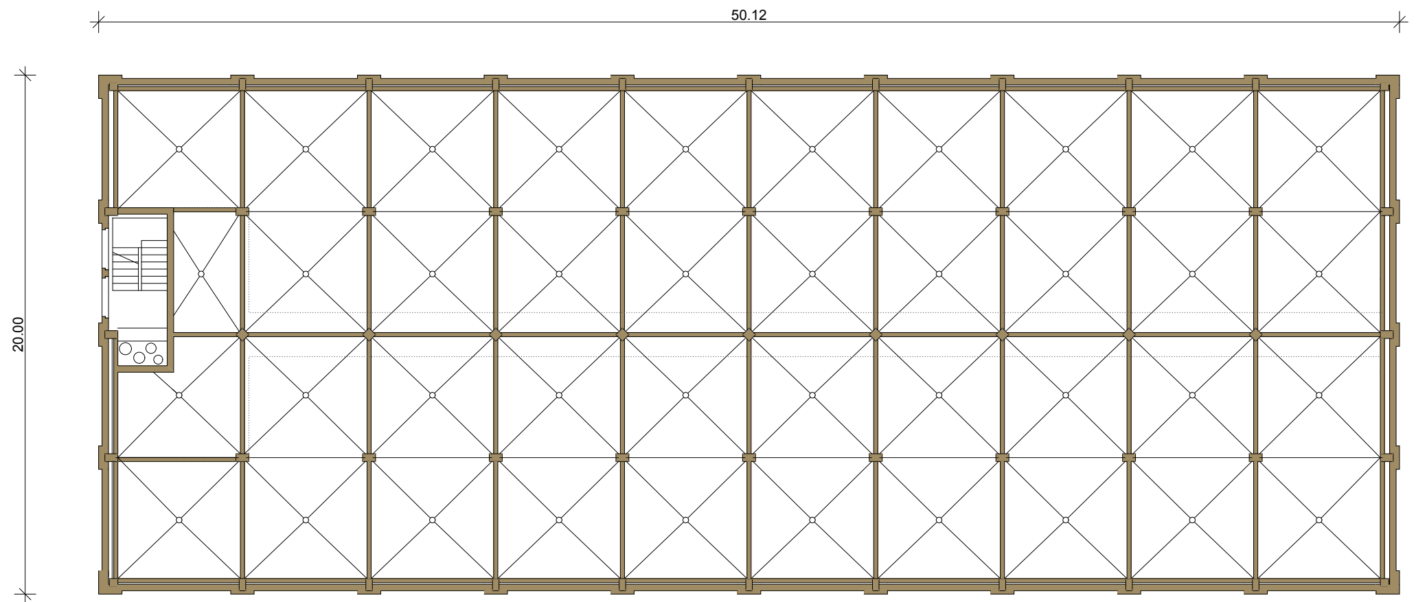
1. Obergeschoss Silogebäude (+5.54)
