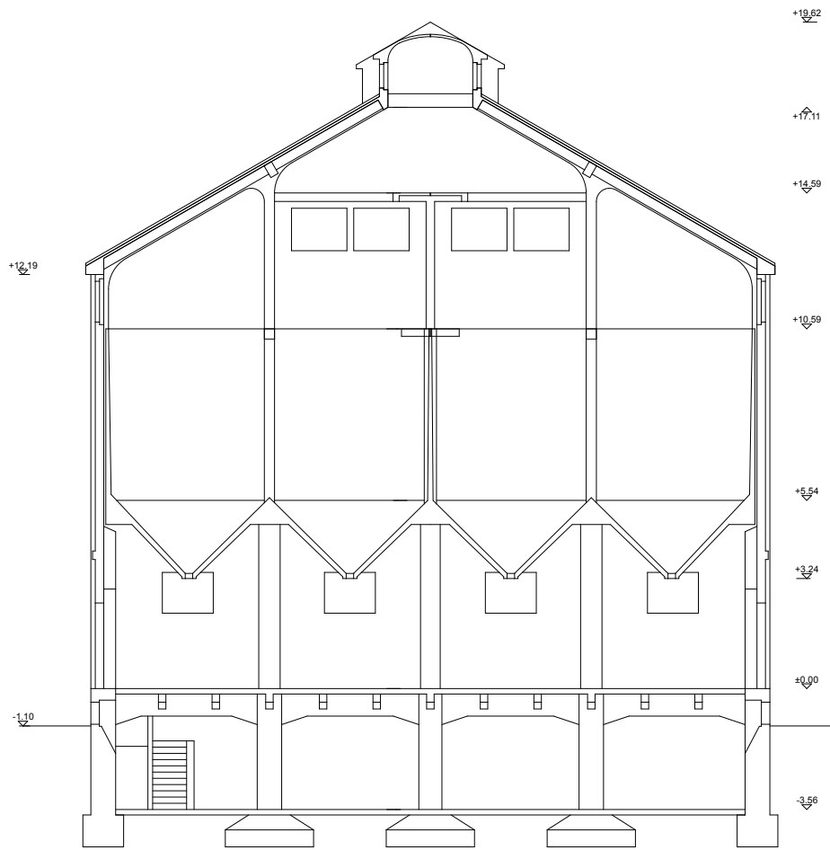
Querschnitt Silogebäude
