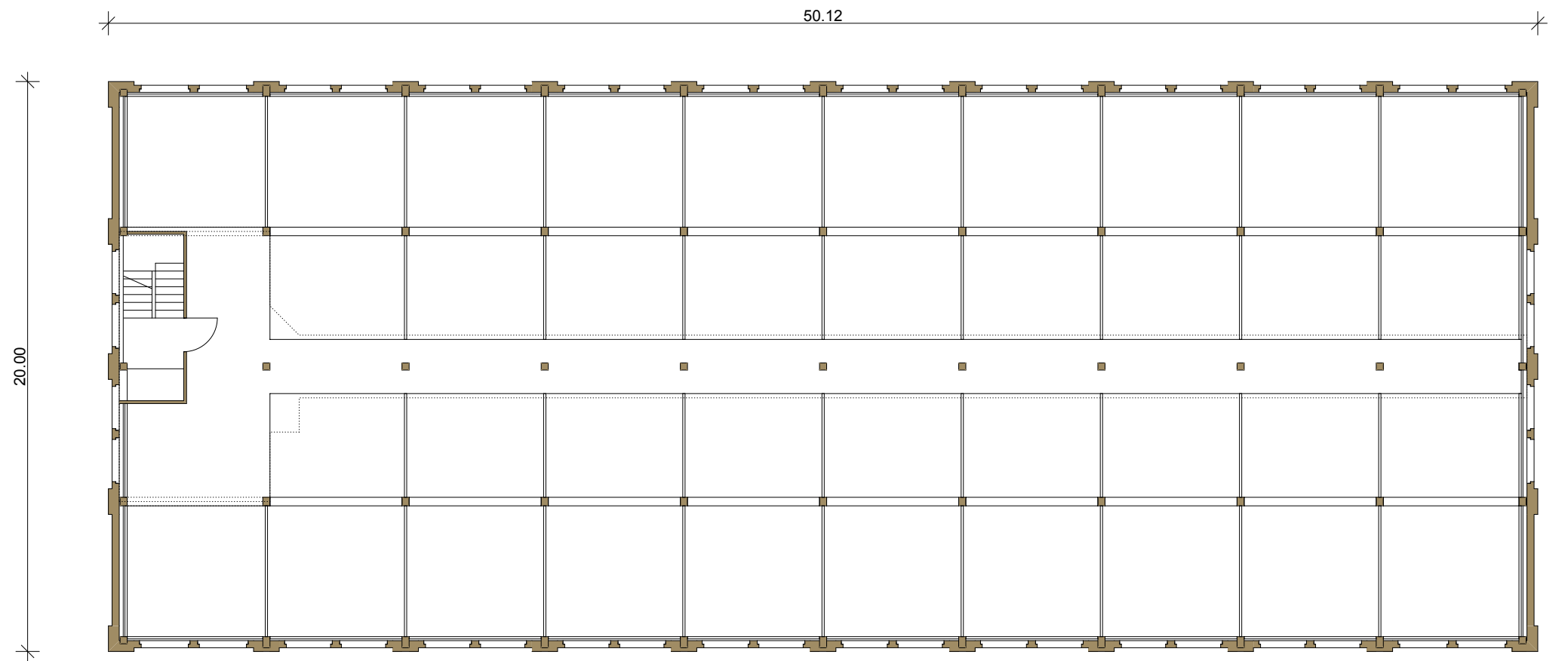
2. Obergeschoss Silogebäude (+10.59)
